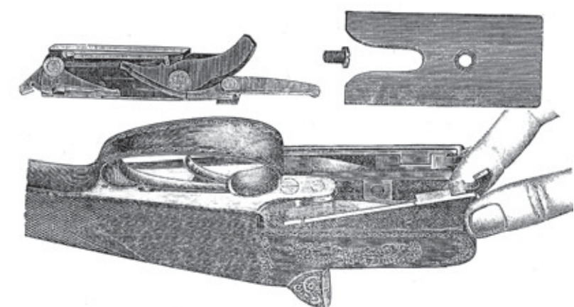
Так выглядел первый дропlock. Рисунок из каталога Вестли Ричардс 1898 г.
