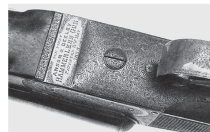
Замок модели Франкотта №24, выполненный Филиппом Бернтхейзелом из Люневилля (слева). Первый бокlock (справа)
